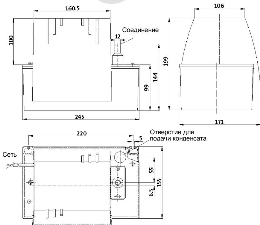
Рис. 2 Габаритный чертеж
