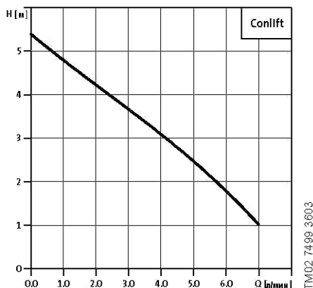
Рис. 9 График характеристики
