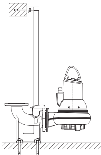
Рис. 4 Погружная установка на автоматической трубной муфте
