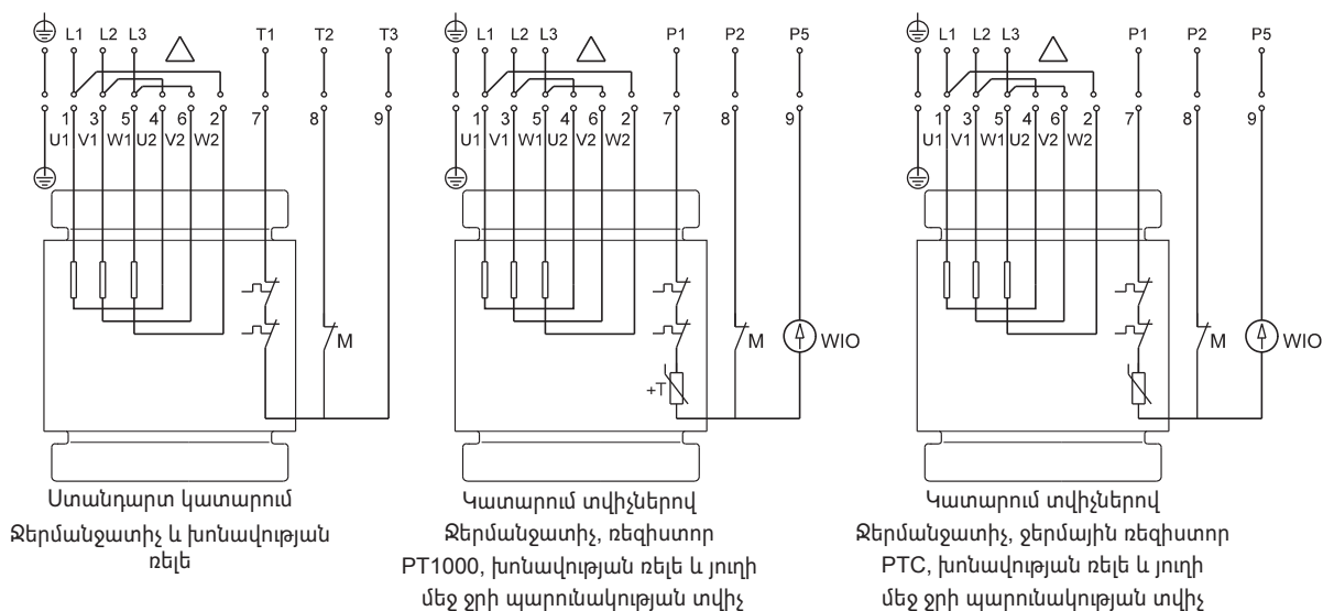
Նկար 9 10-ջիղանի մալուխի համար էլեկտրական միացումների սխեմա, միացում ,եռանկյունի (D)
