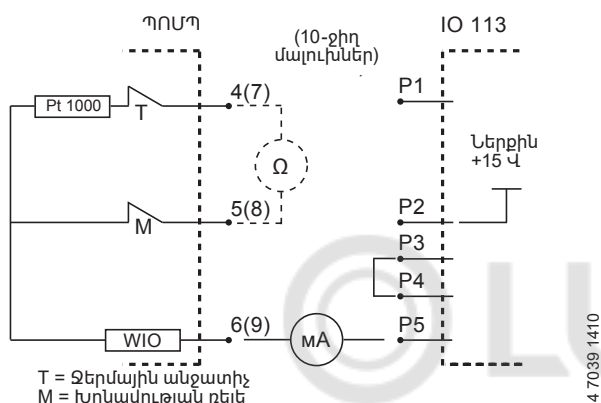
Նկար 16 Pt1000-ով SE1 և SEV պոմպեր
