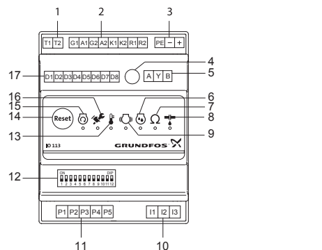
Նկար 15 Մոդուլ IO 113
