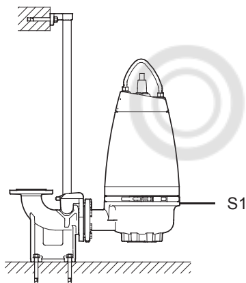
Նկար 20 Ավտոմատ խողովակային ագույցի վրա տեղադրման ընկերմիտ տեսակ:
