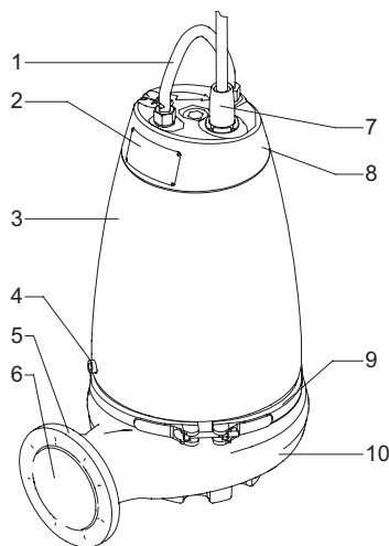
1-сүр. SE соркымасы
