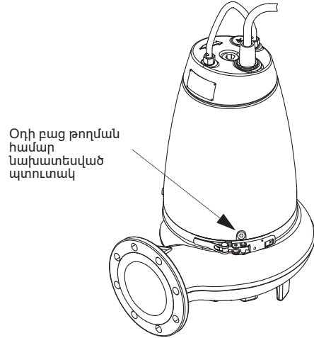
Նկար 18 Օդի բաց թողման համար նախատեսված պոմպի մարմին
