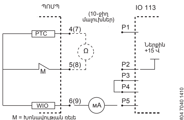
Նկար 17 Pt1000 տվիչով SE1 և SEV պոմպեր
