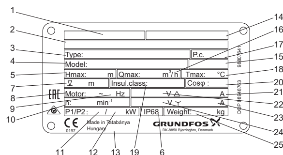
Рис. 2 Фирменная табличка
