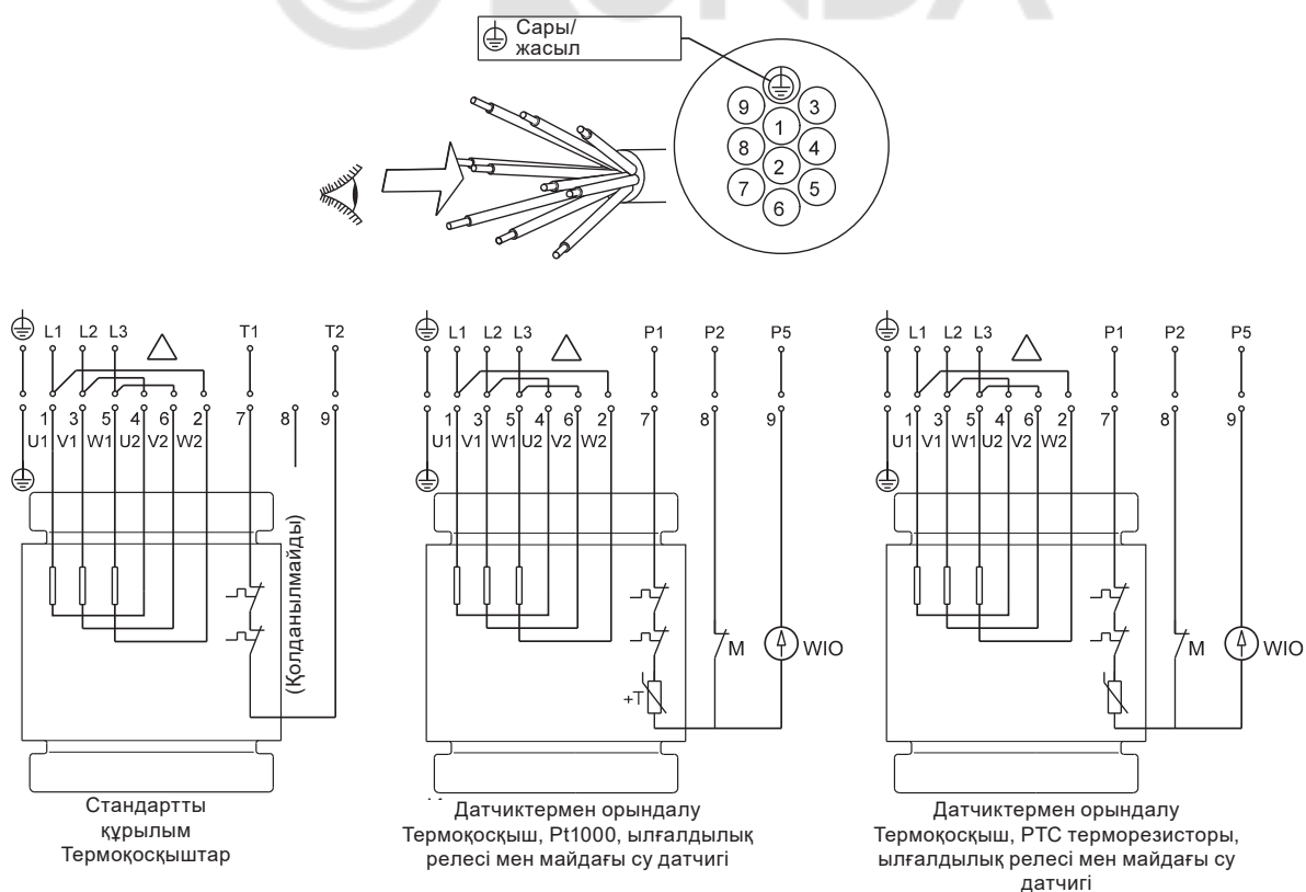
12-сур. 10-тарамдық кабель үшін электр қосылыстардың схемасы, «үшбұрыш» (D) қосылысы
