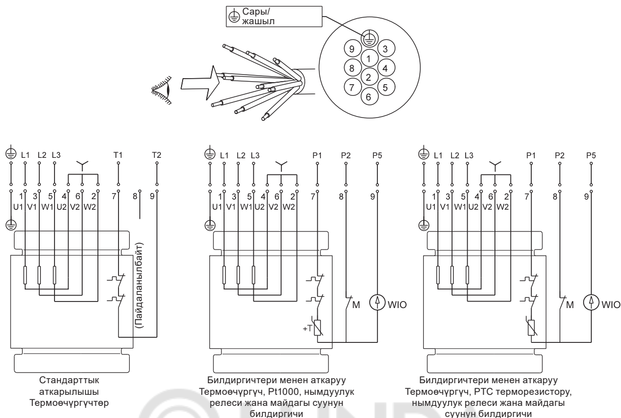
11-сүр. 10 зымдуу кабель үчүн электрдик байланыштардын схемалары, «жылдыз» (Y)
