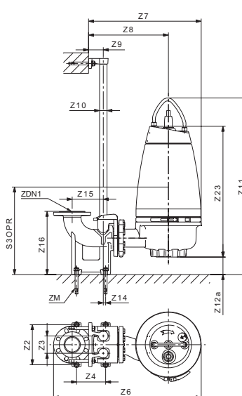
Рис. 33 Насос SEV
