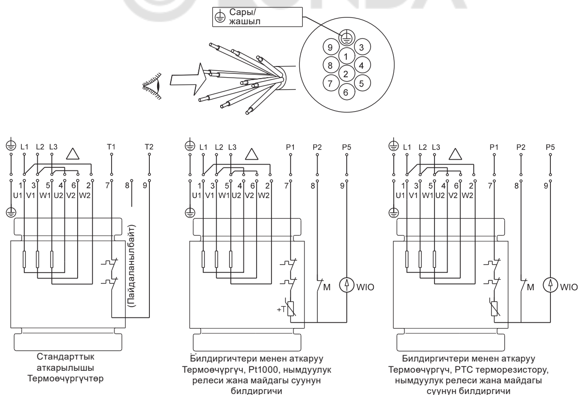
12-сүр. 10 зымдуу кабель үчүн электрдик байланыштардын схемасы, «үч бурчтук» (D)
