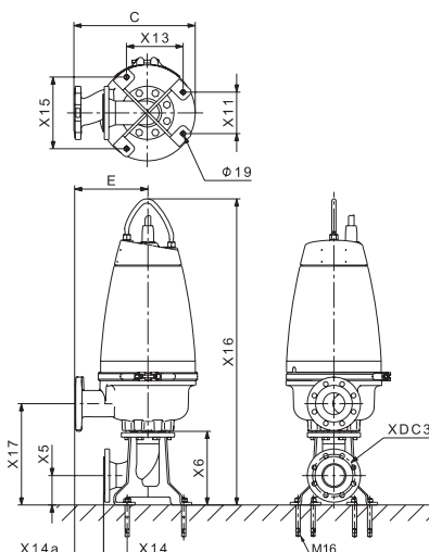
Рис. 37 Насос SEV
