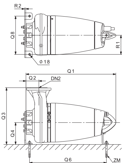
Рис. 34 Насос SE1
