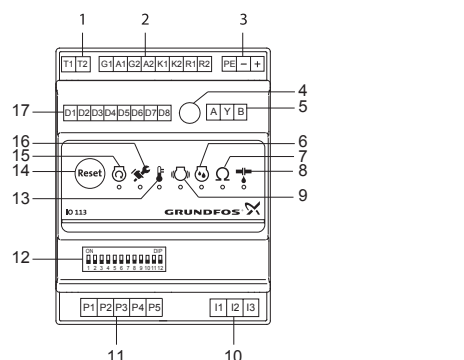
15-сүр. IO 113 модулу
