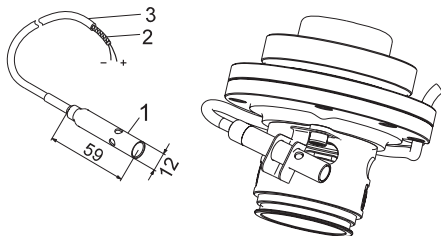
Նկար 14 Տվիչ WIO
