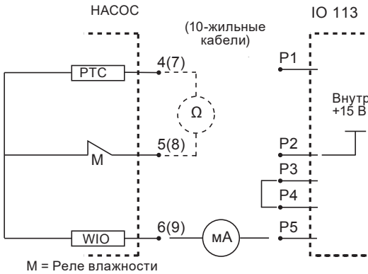
Рис. 17 Насосы SE1, SEV с датчиком PTC
