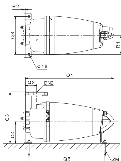
Рис. 35 Насос SEV
