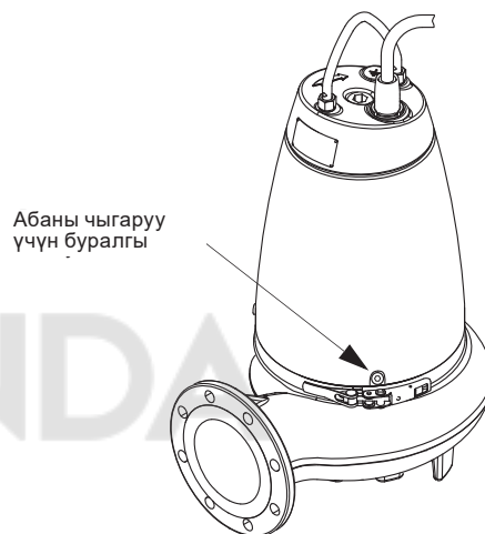
18-сүр. Абаны чыгаруу үчүн буралгы
