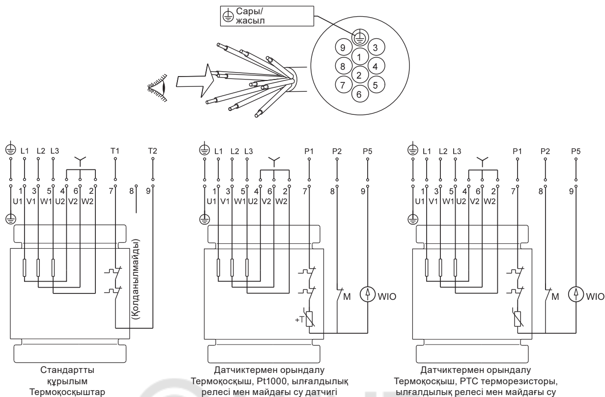
11-сур. 10-тарамдық кабель үшін электр қосылыстардың схемасы, «жұлдызша» (Y) қосылысы
