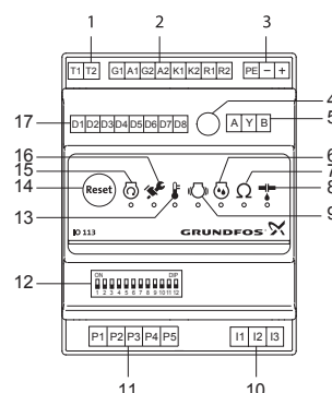
Рис. 15 Модуль IO 113
