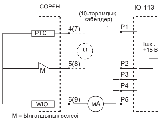
17-сұр. РТС датчигімен SE1, SEV сорғылары
