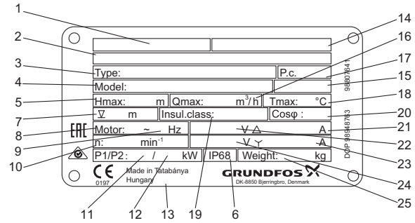
Նկար 2 Ֆիրմային վահանակ
