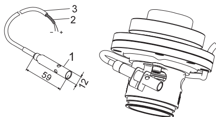
Рис. 14 Датчик WIO
