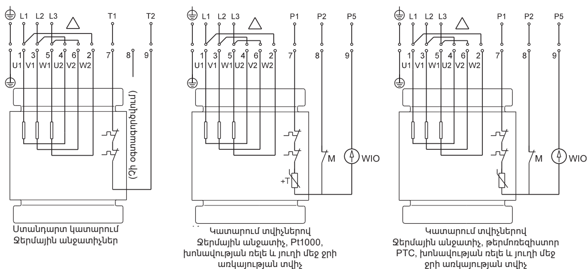
Նկար 12 Էլեկտրական միացումների սխեմաները 10 ջիլ մալուխի համար, միացում «եռանկյուն» (D)
