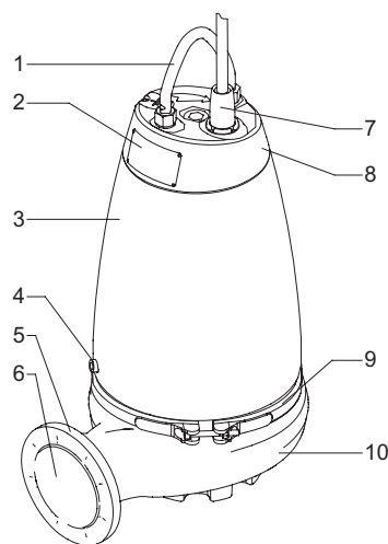
Рис. 1 Насос SE
