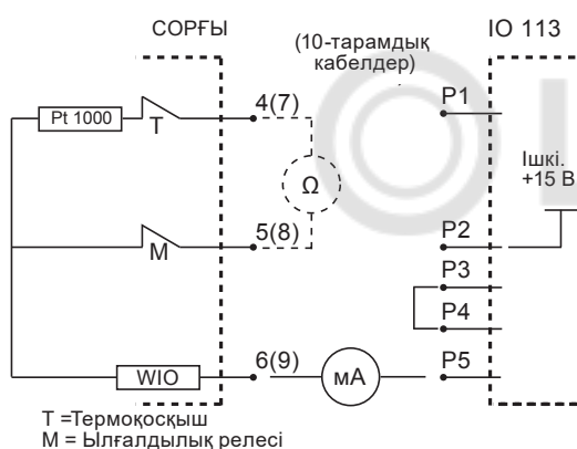
16-сүр. Pt1000-мен SE1, SEV сорғылары
