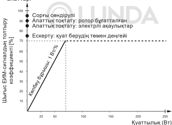
15-сур. Кері байланыс ЕИМ-сигналының бейіні
