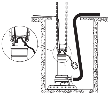
4-сүр. Соркысманы резервуардан көтөрүүнүн мисалы
