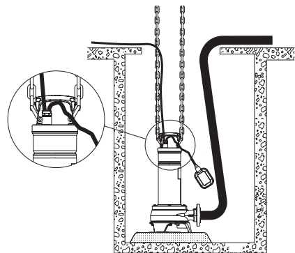
Նկար 4 Ռեզերվուարից պոմպը բարձրացնելու օրինակ
