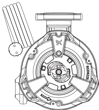
Рис. 11 Проверка вращения рабочего колеса
