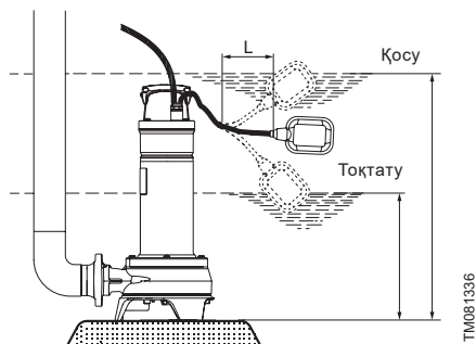
8-сур. Қалтқылы ажыратқыштың күйін реттеу
