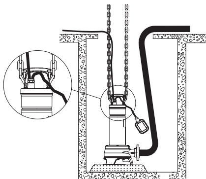
Рис. 4 Пример подъема насоса из резервуара
