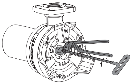
Рис. 14 Снятие режущей головки
