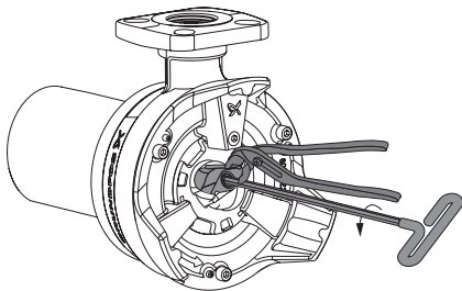
Նկար 14 Կտրող գլխիկի հեռացում
