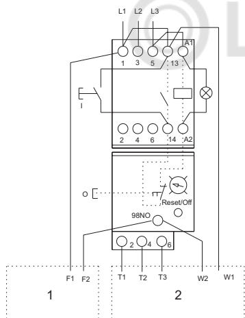
9-сүр. Үч фазалуу кыймылдаткычтын электрдик схемасы, мында 1 - калкыма өчүргүч, 2 - электр кыймылдаткычы
