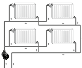
Рис. 30 Двухтрубная система отопления
