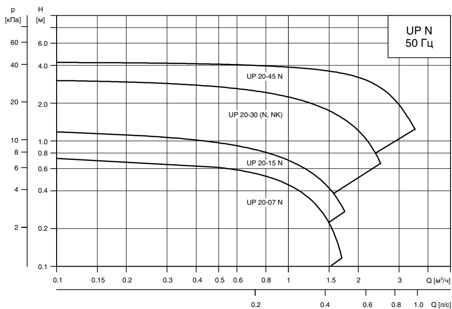
Рис. 27 Расходно-напорная характеристика насосов UP N
