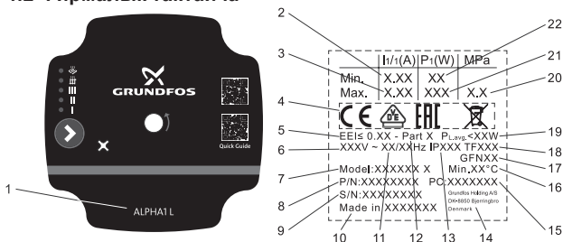
1-сүр. ALPHA1 L соркысмасынын фирмалык көрнөкчөсү
