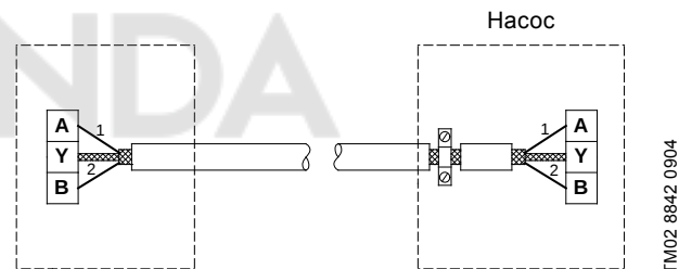
Рис. 18 Подключение 2-жильного экранированного кабеля
