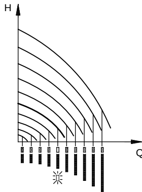
Рис. 28 Настройка производительности насоса в нерегулируемом режиме
