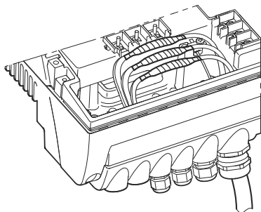
Рис. 44 Изолированные провода
