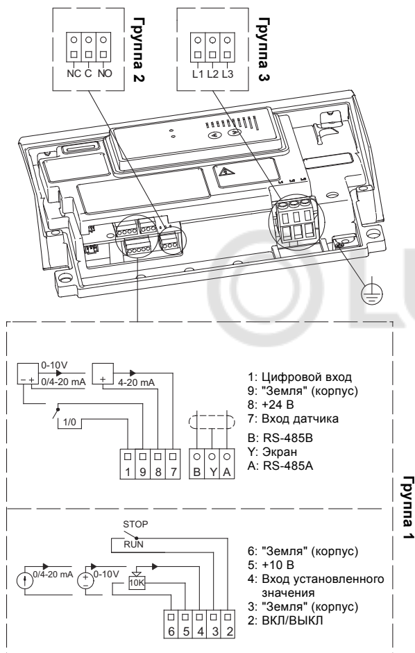
Рис. 8 Клеммы насосов TPE, NKE, NKGE и NBE, NBGE
