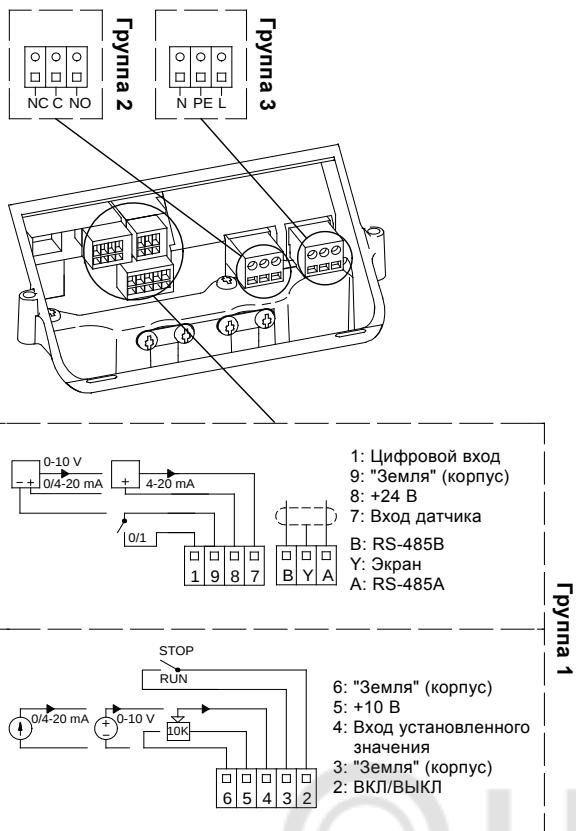
Рис. 4 Клеммы насосов TPE, NKE, NKGE и NBE, NBE
