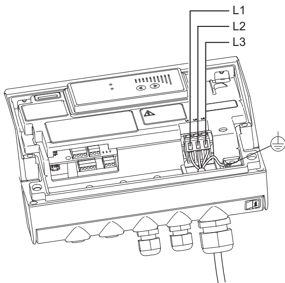
Рис. 7 Подключение электропитания
