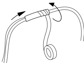
Рис. 43 Изоляция проводов
