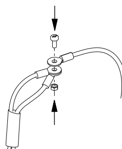
Рис. 42 Подключение проводов
