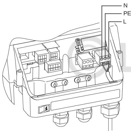
Рис. 3 Подключение электропитания
