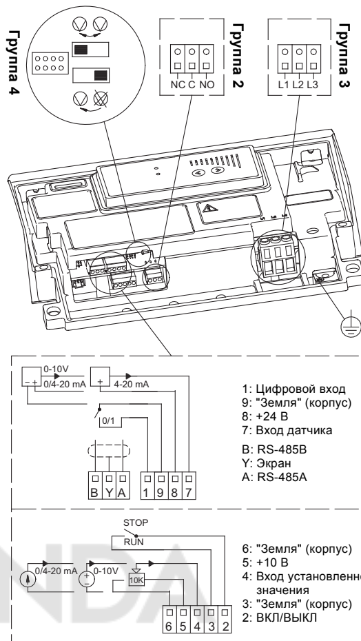
Рис. 9 Клеммы насосов TPED
