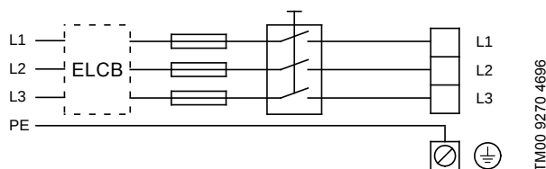
Рис. 10 Подключенный к сети насос с сетевым выключателем, плавкими предохранителями, дополнительной защитой и защитным заземлением
