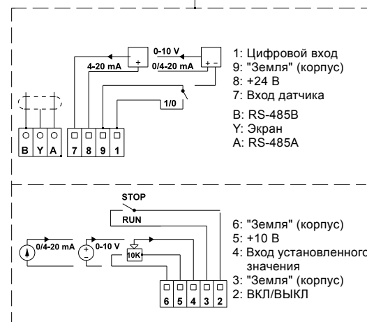
Рис. 14 Клеммы насосов TPE, NKE, NKGE и NBE, NBGE
