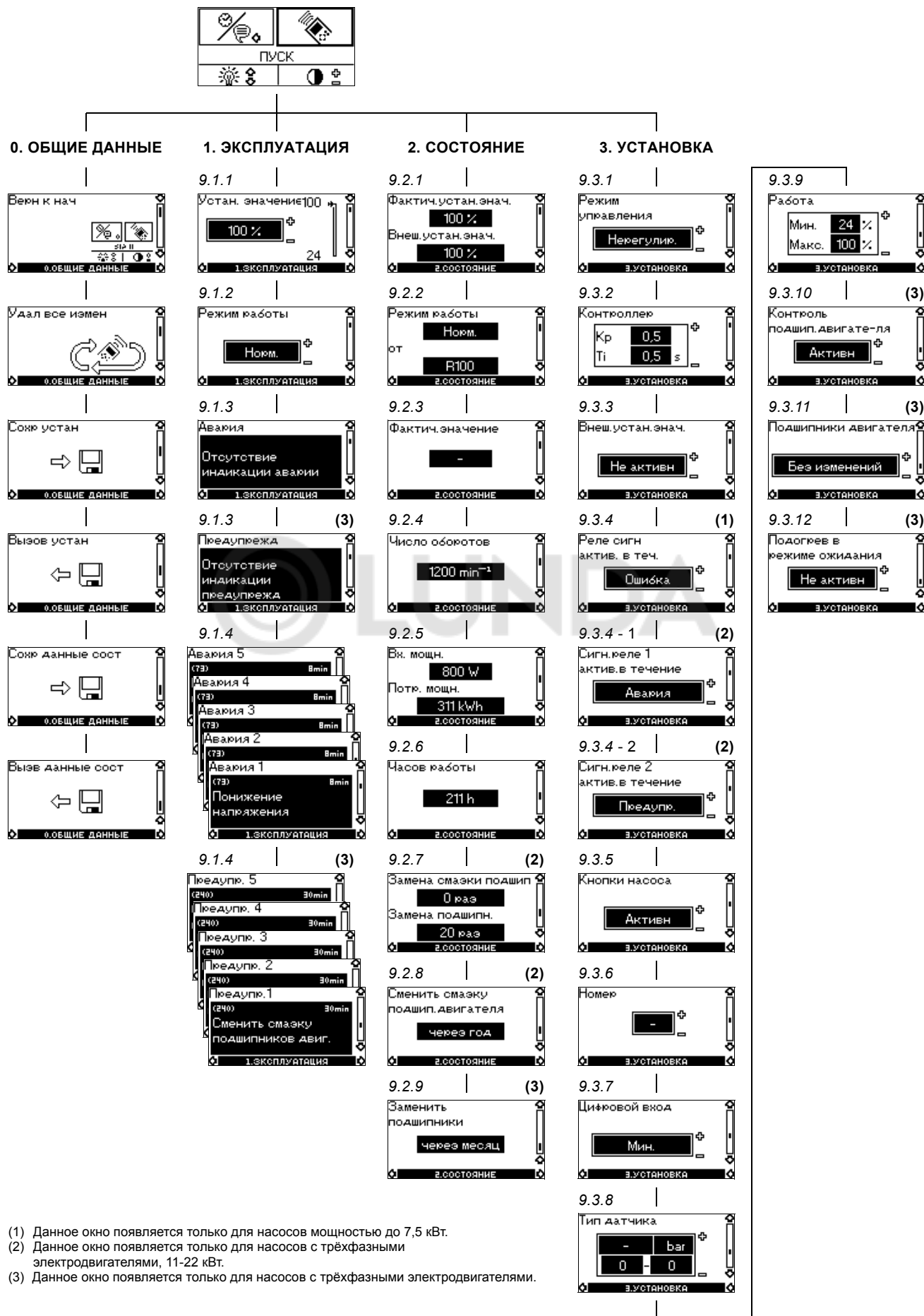
Рис. 32 Обзор меню
