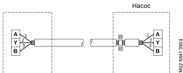
Рис. 17 Подключение 3-жильного экранированного кабеля
