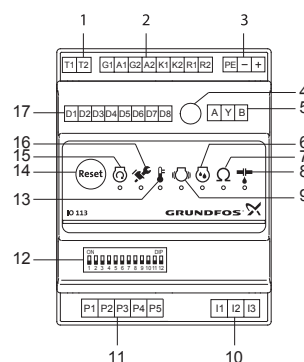
Рис. 15 Модуль IO 113
