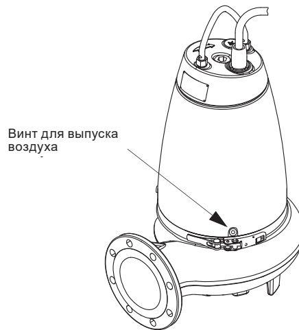
Рис. 18 Винт для выпуска воздуха
