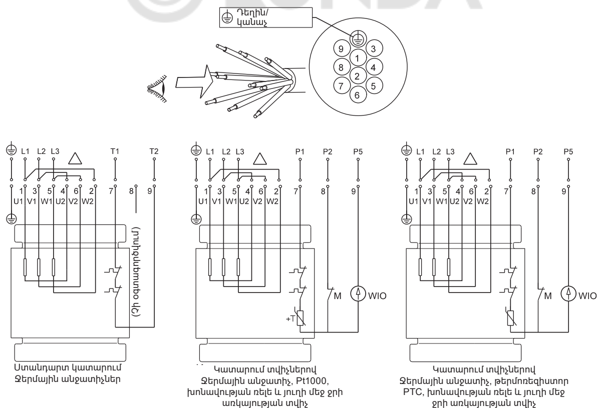
Նկար 12 Էլեկտրական միացումների սխեմաները 10 ջիլ մալուխի համար, միացում «եռանկյուն» (D)
