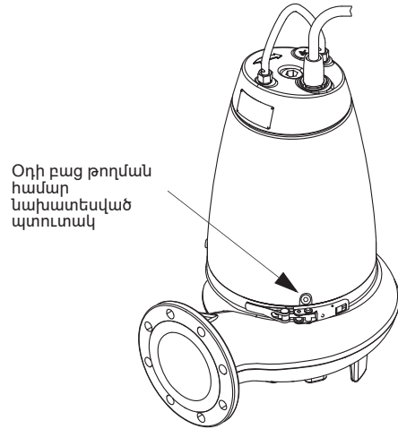
Նկար 18 Օդի բաց թողման համար նախատեսված պոմպի մարմին
