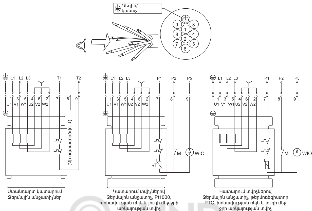
Նկար 11 Էլեկտրական միացումների սխեմաները 10 ջիլ մալուխի համար, միացում «աստղ» (Y)
