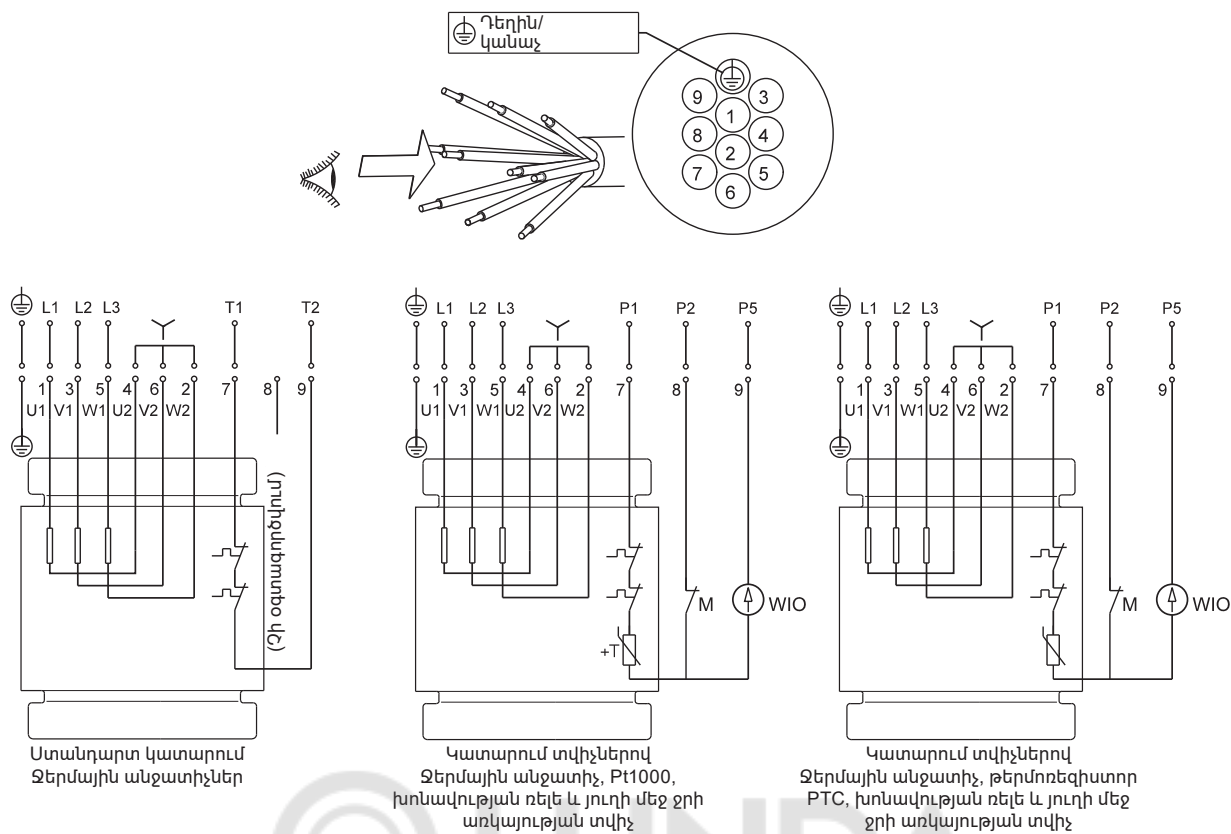
Նկար 11 Էլեկտրական միացումների սխեմաները 10 ջիղ մալուխի համար, միացում «աստղ» (Y)
