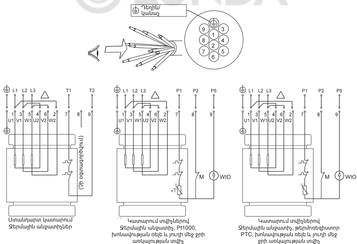
Նկար 12 Էլեկտրական միացումների սխեմաները 10 ջիղ մալուխի համար, միացում «եռանկյուն» (D)
