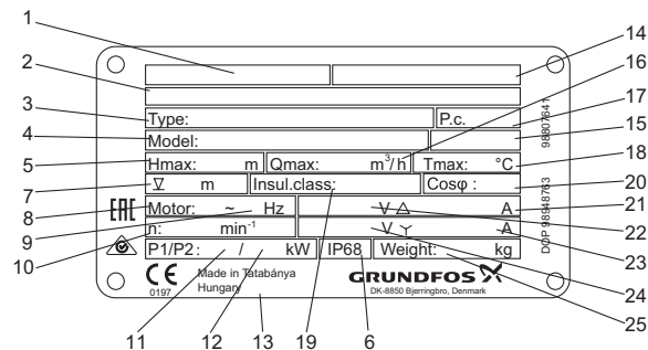
Рис. 2 Фирменная табличка
