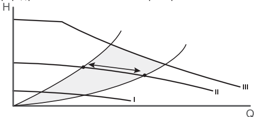
14-сүр. Соркысманын II-белгиленген ылдамдыкта иштеп жатканда тутумдун чыгымдык-кысымдык мүнөздөмөсүнүн мисалы
