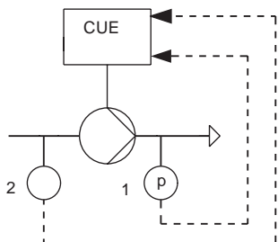
Рис. 90 Перепад давления от двух датчиков
