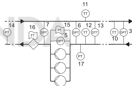
Рис. 24 Отопление и охлаждение, насосы в обратном трубопроводе
