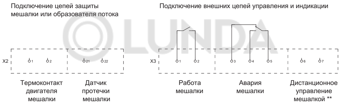
Рис. 70 Подключение сигнальных цепей
