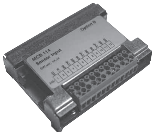
Рис. 141 Модуль расширения входов MCB 114
