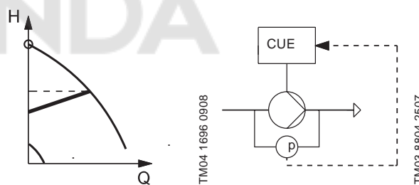
Рис. 93 Пропорциональный перепад давления, обновление H макс.
