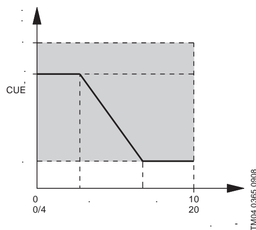
Рис. 103 Сокращенный обратный сигнал внешнего установленного значения.
