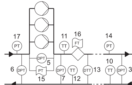
Рис. 23 Отопление и охлаждение, насосы в подающем трубопроводе
