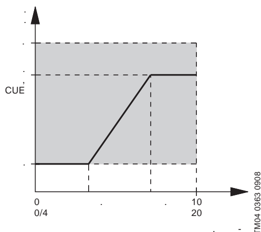
Рис. 101 Сокращенный сигнал внешнего установленного значения
