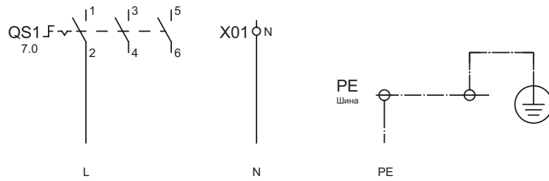
Рис. 45 Подключение питающей сети для однофазных шкафов.
