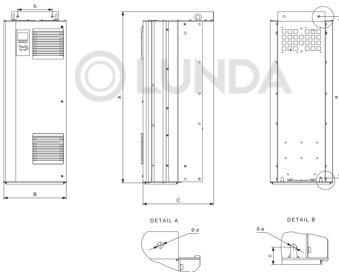
Рис. 138 Корпусы D1h и D2h
