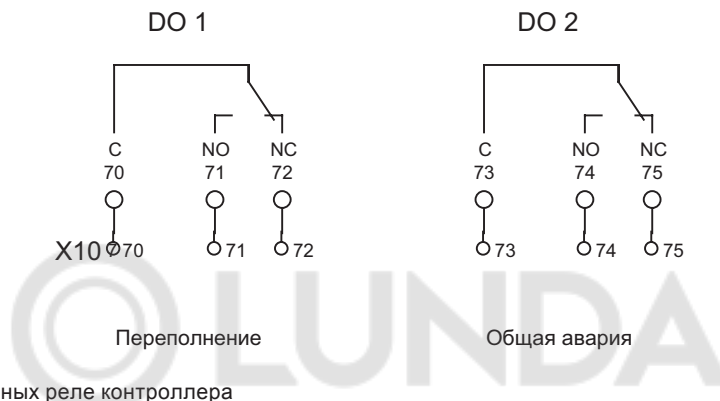
Рис. 67 Выводы сигнальных реле контроллера
