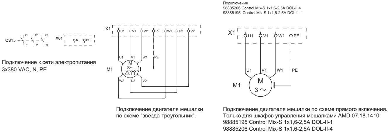
Рис. 69 Подключение силовых цепей
