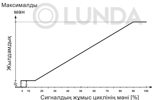
16-сур. ALPHA SOLAR-ға кіріс ЕИМ-сигналдың «С» бейіні
