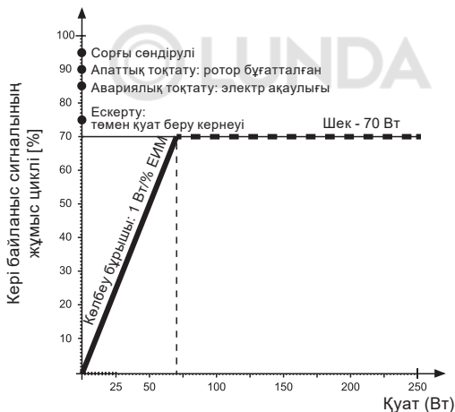
17-сур. Кері байланыс ЕИМ-сигналының бейіні
