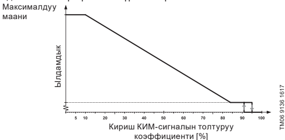
14-сүр. ALPHA1 Lги КИМ-сигналды башкаруучунун профили
