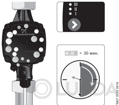
Рис. 10 Удаление воздуха из насоса
