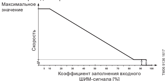
Рис. 14 Профиль управляющего ШИМ-сигнала в ALPHA1 L
