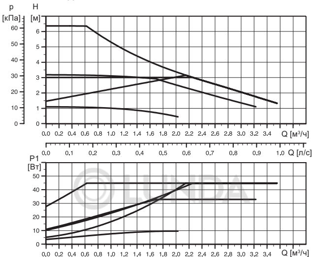
Рис. 18 Расходно-напорная характеристика насосов серии ALPHA1 L
