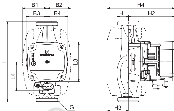
Նկար 17 Գաբարիտային չափեր
