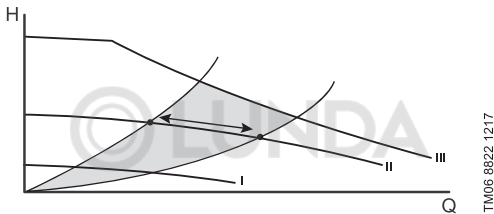
Նկար 13 Ֆիքսված արագությունների երեք կորերի օրինակ
