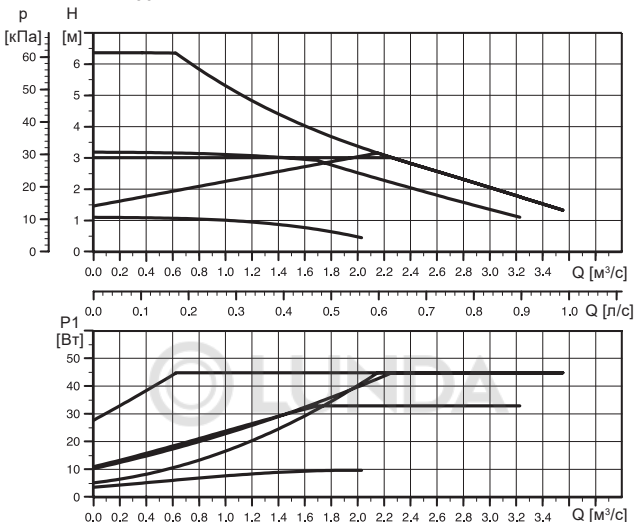
18-сүр. ALPHA1 L сериясынын соркысмаларынын чыгымдык-кысымдык мүнөздөмөсү
