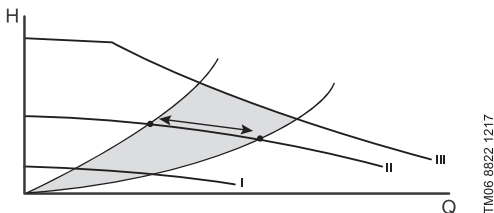
13-сүр. Белгиленген ылдамдыктардын үч ийри сызыгынын мисалы
