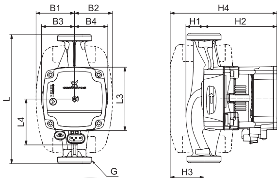
Рис. 19 Габаритные размеры
