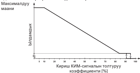
14-сүр. ALPHA1 Lги КИМ-сигналды башкаруучунун профили
