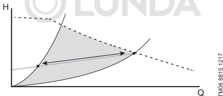
12-сур. Пропорционалдық қысым режимінде қысық пропорционалдық қысымның мысалы
