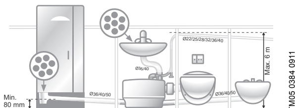
Рис. 23 Пример монтажа
