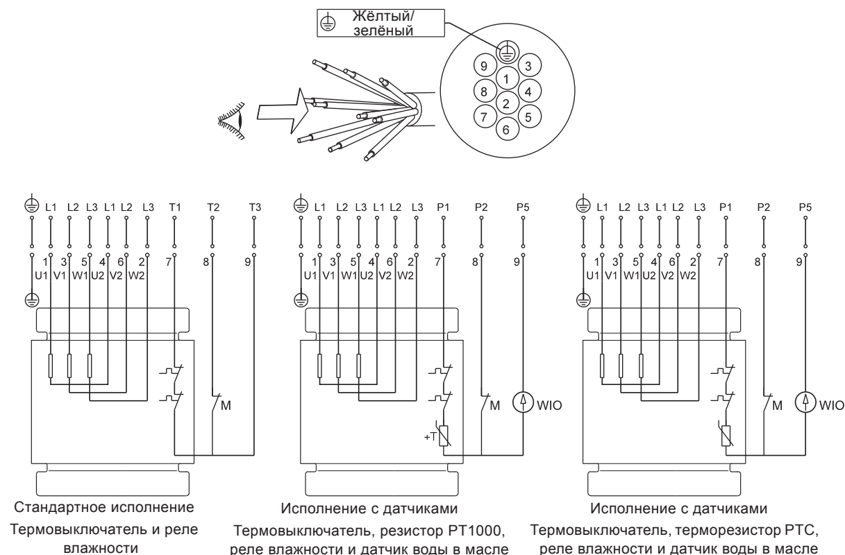
Рис. 7 Схемы электрических соединений для 10-жильного кабеля, соединение «звезда-треугольник» (Y/D)
