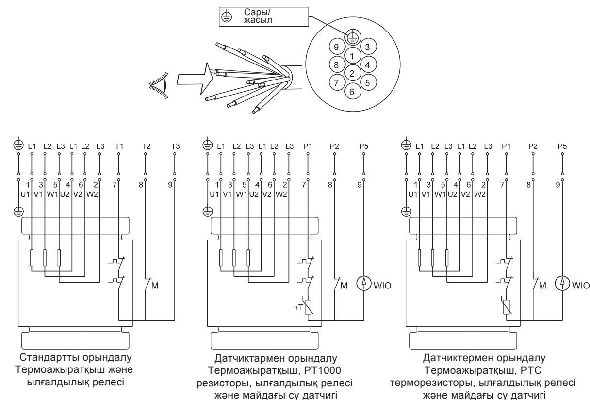
7-сур. 10-тармақты кабельге арналған электр жалғаулар схемасы, «жұлдызша-үшбұрыш» жалғауы (Y/D)
