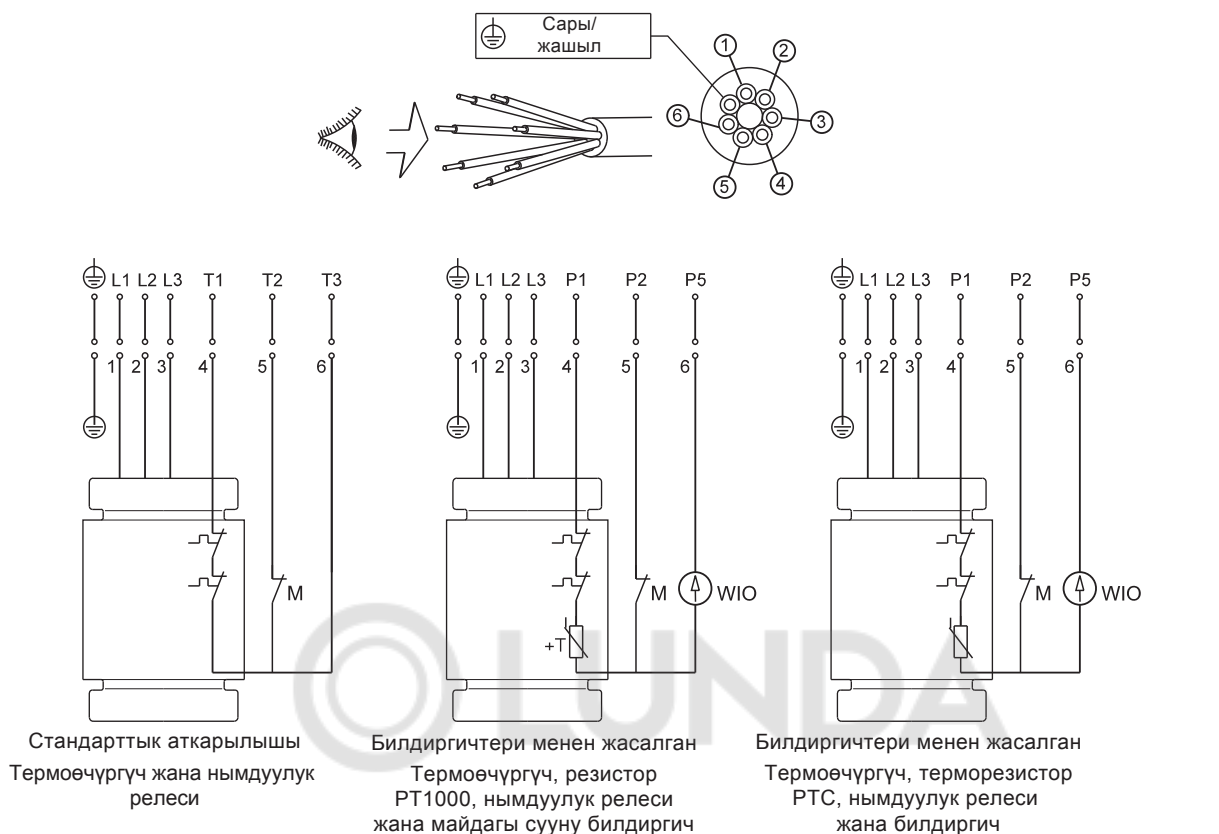
Сүр. 6 7-катмарлуу кабели үчүн электр туташуулардын түзмөктөрү, түз иштетүү
