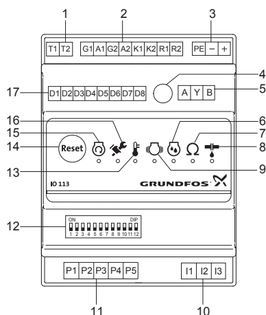
Сүр. 11 IO 113 модуль
