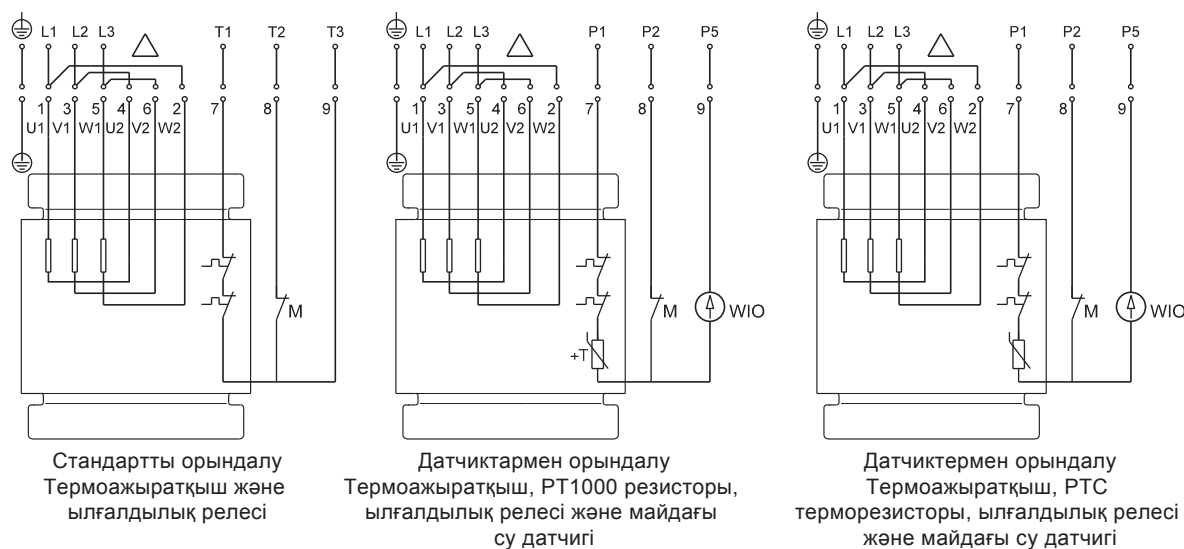
9-сур. 10-тармақты кабельге арналған электр жалғаулар схемасы, «үшбұрыш» жалғауы (D)
