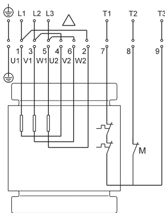
Стандарттык аткарылышы Термоөчүргүч жана нымдуулук релеси
