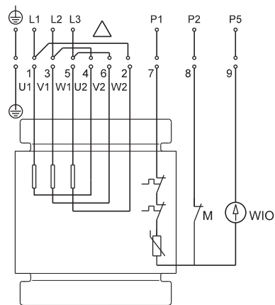
Билдиргичтери менен жасалган Термоөчүргүч, терморезистор PTC, нымдуулук релеси жана билдиргич
