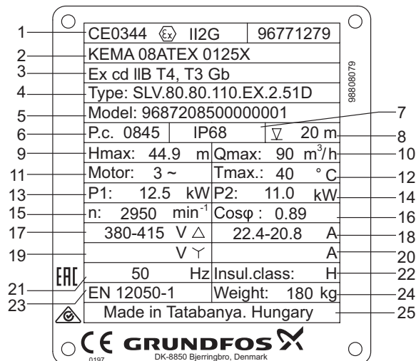
Рис. 2 Фирменная табличка
