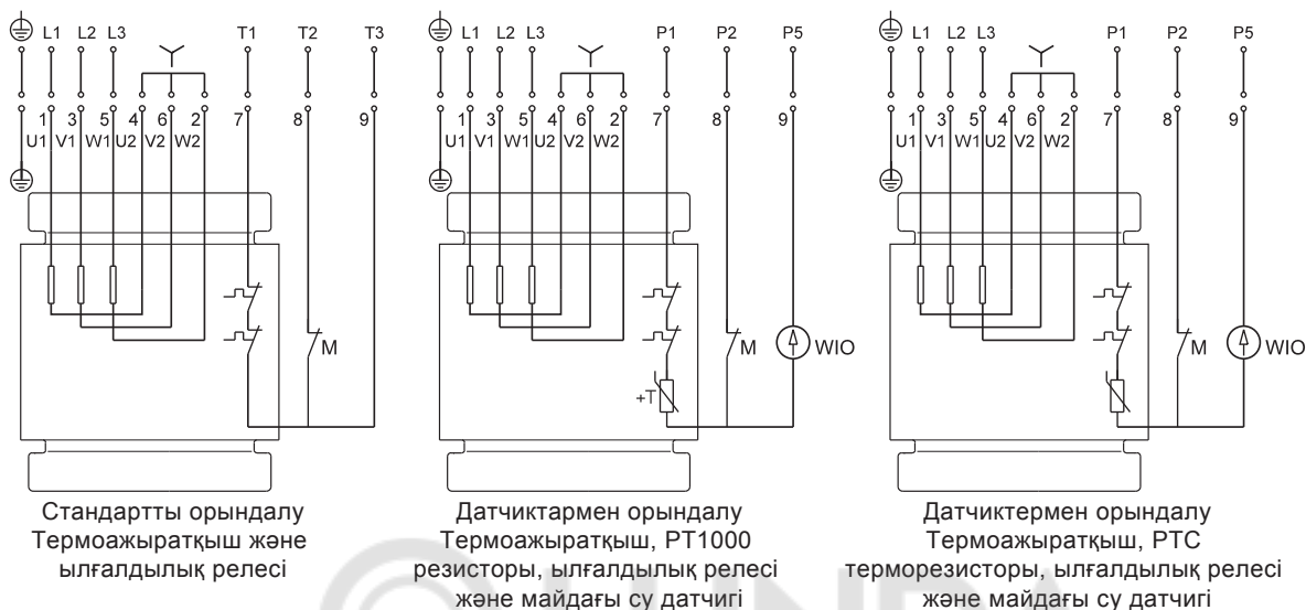
8-сур. 10-тармақты кабельге арналған электр жалғаулар схемасы, «жұлдызша» жалғауы (Y)
