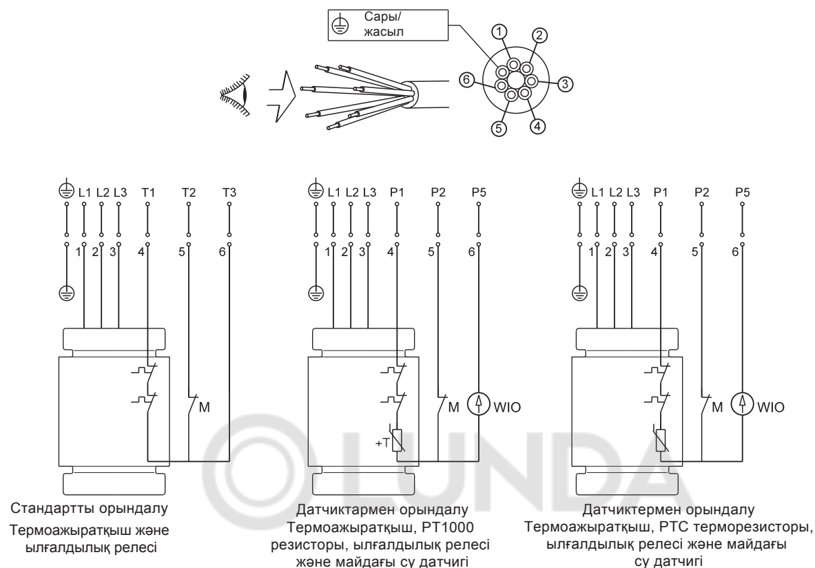
6-сур. 7-тармақты кабельге, арналған электр жалғауларының схемасы, тікелей іске қосу
