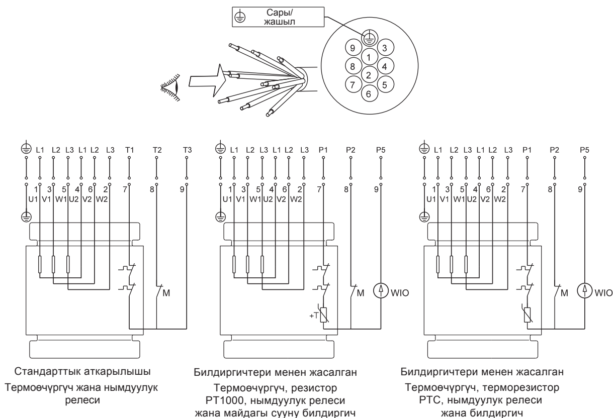
Сүр. 7 10-катмарлуу кабели үчүн электр туташуулардын түзмөктөрү, «жылдыз-үч бурчтук» туташуу (Y/D)
