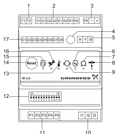
Рис. 11 Модуль IO 113
