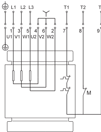
Стандарттык аткарылышы Термоөчүргүч жана нымдуулук релеси
