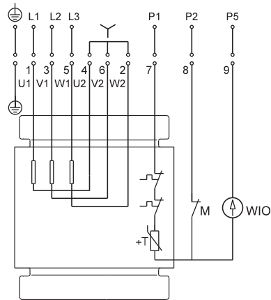
Билдиргичтери менен жасалган Термоөчүргүч, резистор PT1000, нымдуулук релеси жана майдагы сууну билдиргич
