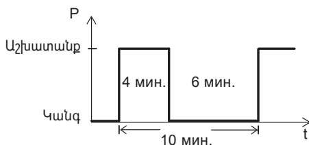
Նկար 14 S3, ընդհատումներով աշխատանք
