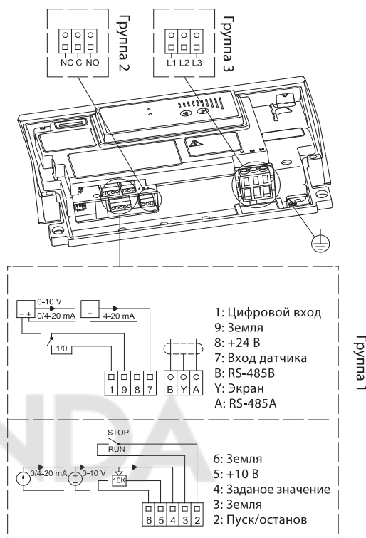
Рис. 37 Схема подключения
