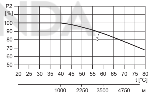
Рис. 33. Зависимость между мощностью на валу электродвигателей MGE (P2) и температурой окружающей среды.
