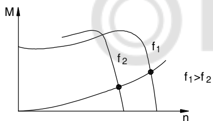
Рис. 42 Смещение характеристики крутящего момента электродвигателя
