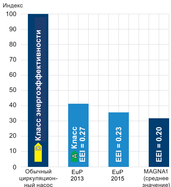
Рис. 24 Индекс энергопотребления
