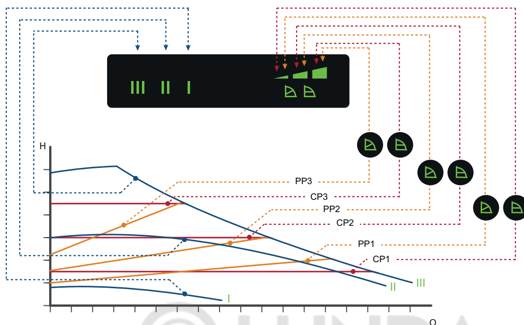
Рис. 20 Режимы управления насоса в зависимости от рабочих характеристик
