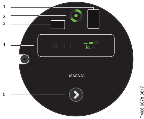
Рис. 21 Панель управления
