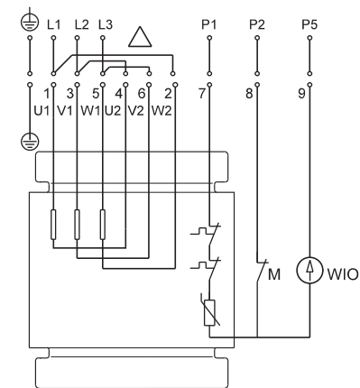
Билдиргичтери менен жасалган Термоөчүргүч, терморезистор PTC, нымдуулук релеси жана билдиргич
