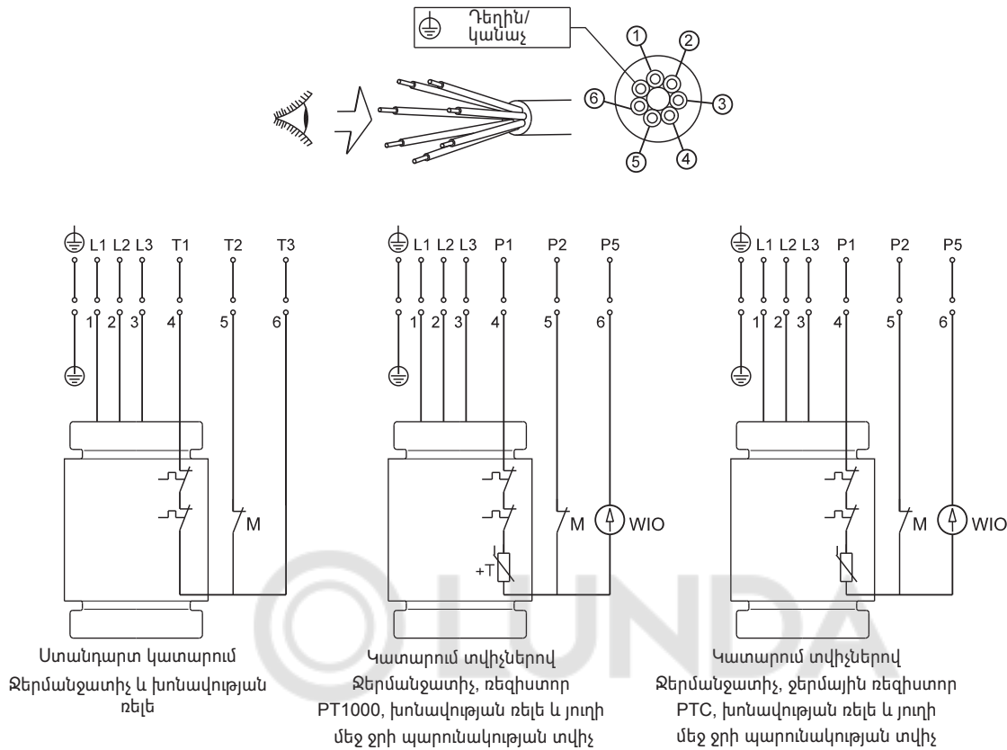
Նկար 6 7-ջիղանի մալուխի համար էլեկտրական միացումների սխեմաներ, ուղղակի մեկնարկ
