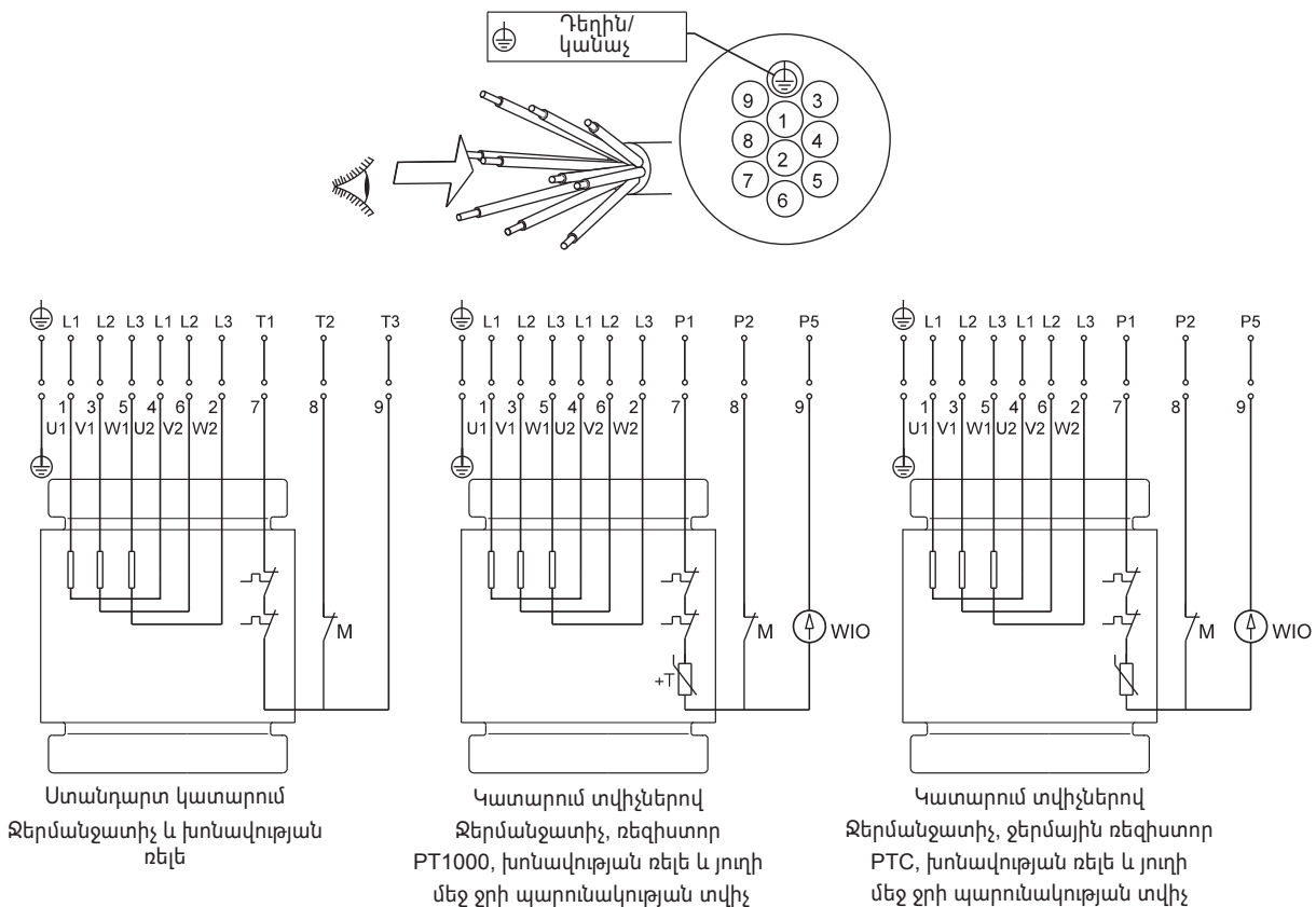
Նկար 7 10-ջիղանի մալուխի համար էլեկտրական միացումների սխեմաներ, միացում, աստղ-եռանկյունի (Y/D)
