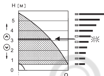
Рис. 18 Установка значения 3 бара, режим регулирования напора
